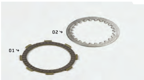
DISQUE D'EMBAYAGE YX YX CLUTCH PLATE 01 ↳ 22330/152FMH (GARNI/ FRICTION) € 6 02 ↳ 22341/152FMH (LISSE/ SMOOTH) € 4
